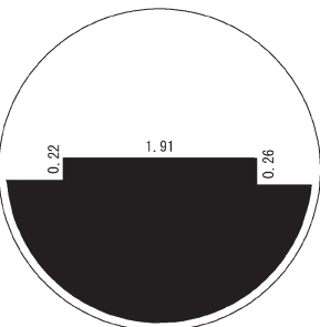
拡大図（ロ）
