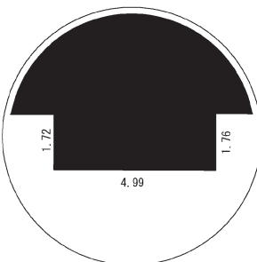
拡大図（ヘ）
