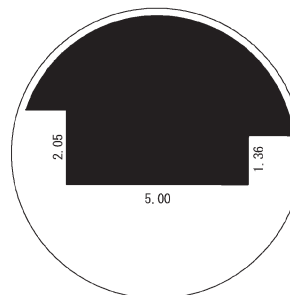
拡大図（チ）
