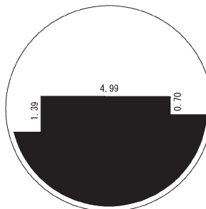
拡大図（ニ）
