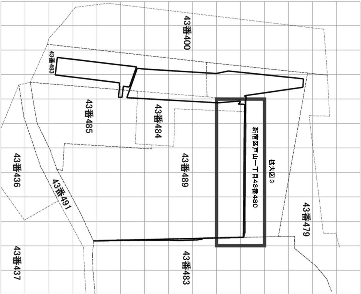
拡大図 2
